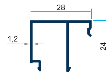
PRV-2174 0.333 gr/m Bim Ç ita
