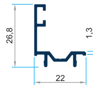
PRV-2175 0.233 gr/m Bim Ç ita
