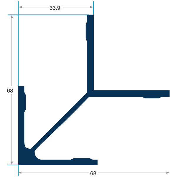
PRV-1150 1327gr/m Yanm Seri Çavuş Köşe
