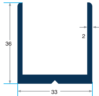
PRV-2080 683gr/m U Profi I
