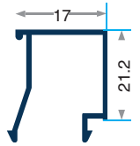
PRV-2050 175gr/m Isı Cam Çıtası 20 mm
