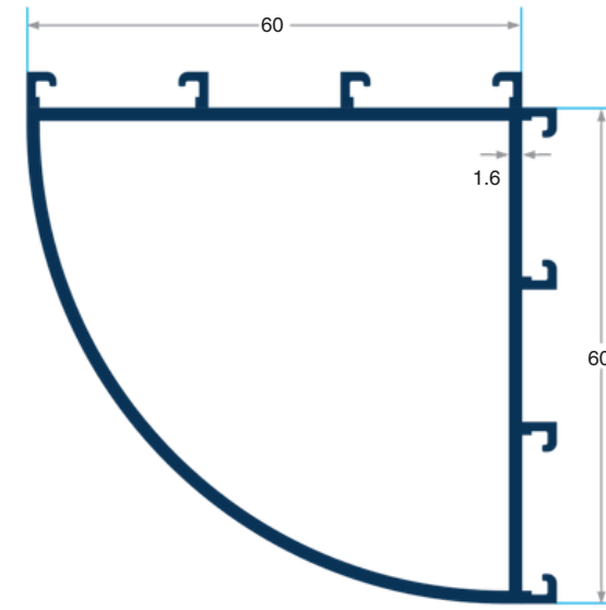
PRV-2150 1133 gr/m Köşe D önuş Profili
