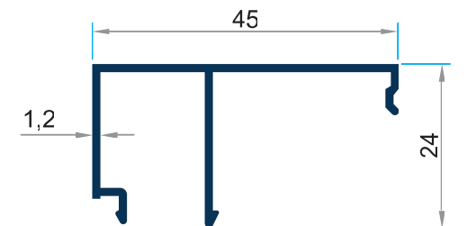
PRV-2173 0.409 gr/m Bim Ç ita
