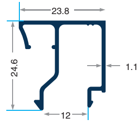
PRV-2061 263gr/m Tek Cam Çıtası 6 mm
