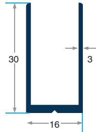
PRV-2070 617 gr/m U Profi I
