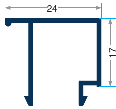
PRV-2060 232gr/m Tek Cam Çıtası 10 mm
