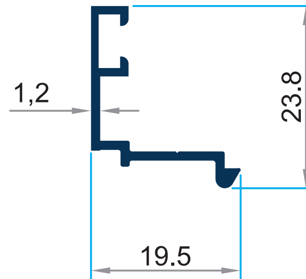
PRV-4354 0.168 gr/m Tırnak Adaptör
