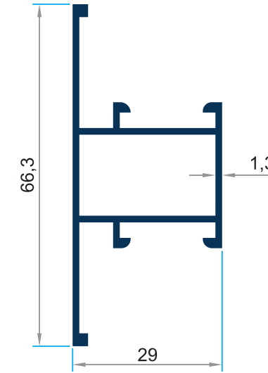
PRV-4351 0.619 gr/m Orta Kayıt Profili
