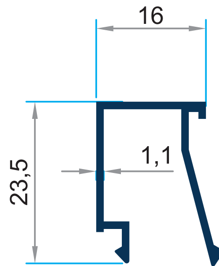
PRV-4353 0.209 gr/m Tek Cam Çıtası
