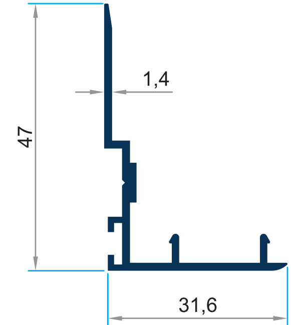
PRV-4352 0.371 gr/m Kenet Profili
