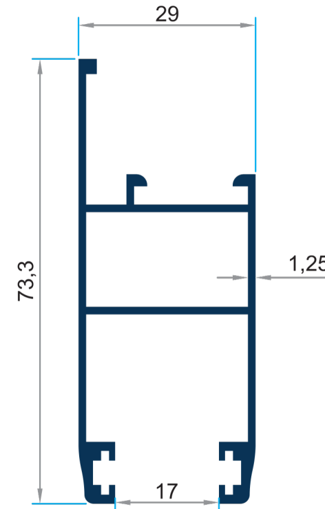
PRV-4350 0.791 gr/m Kanat Profili
