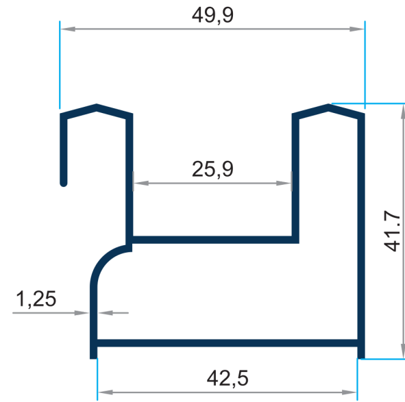
PRV-4355 0.694 gr/m Kasa Profili
