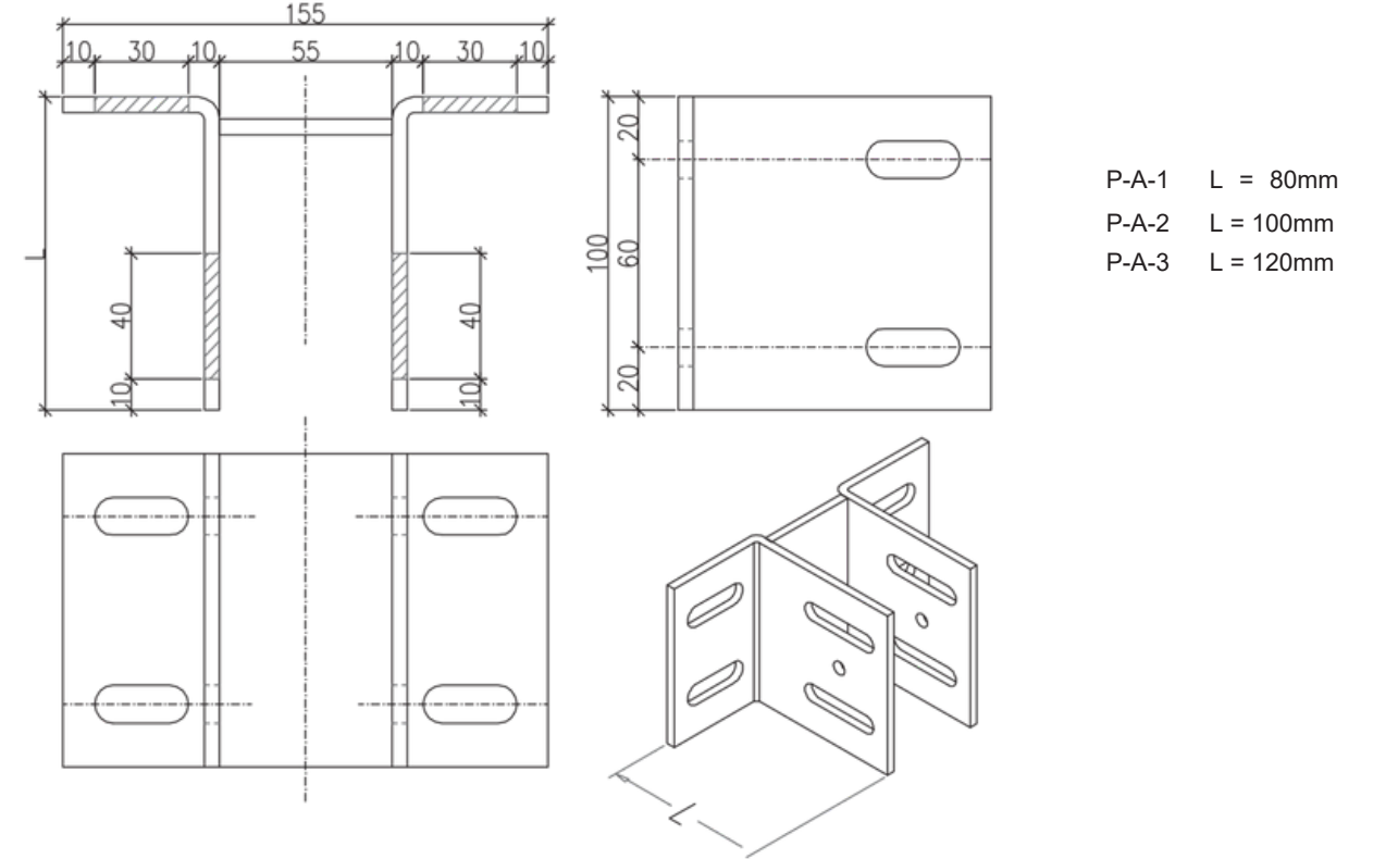
5mm Daldırma Galvanizli Ankraj (Düşey Hareketli)
