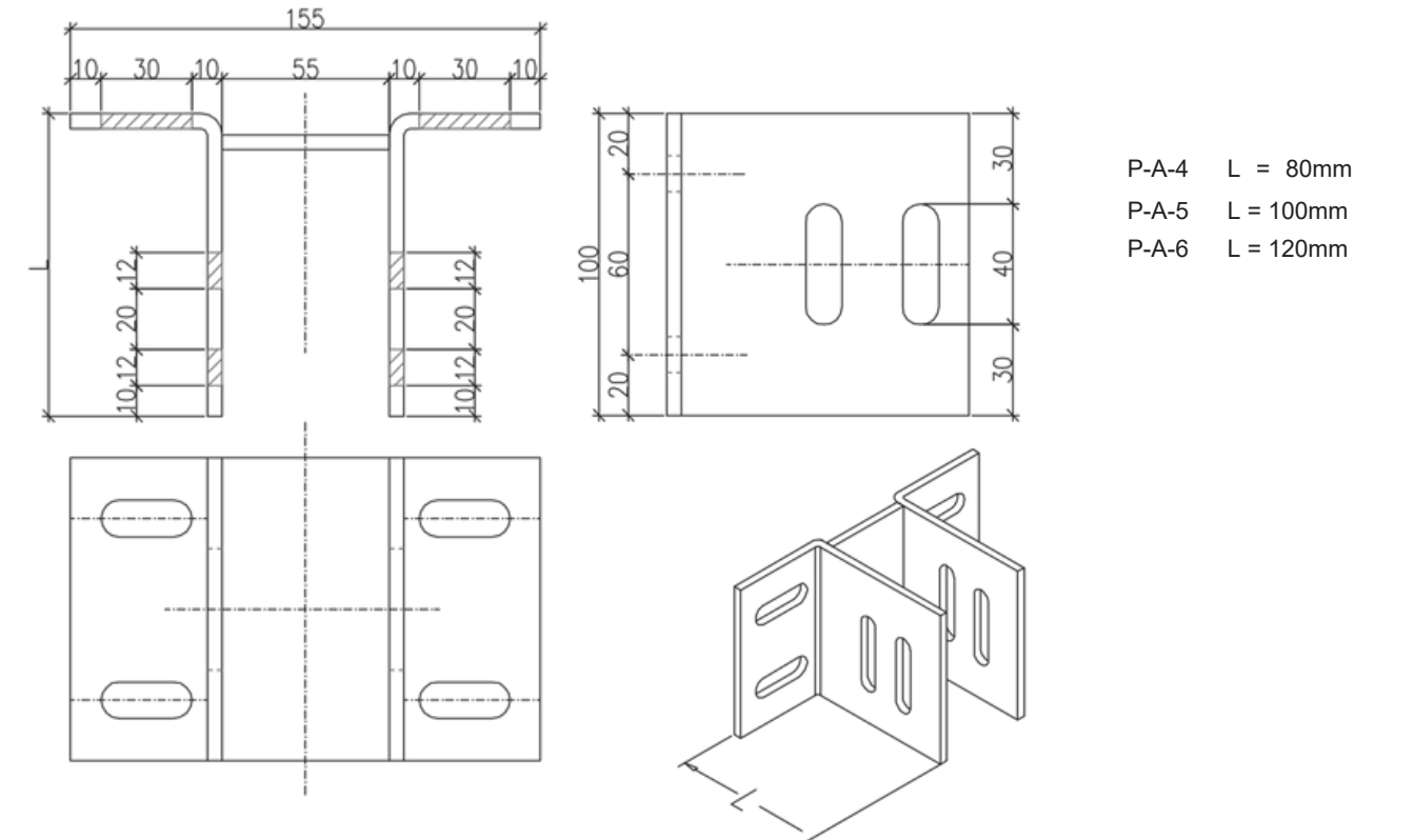
5mm Daldırma Galvanizli Ankraj (Düşey Hareketli)
