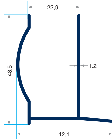
PRV-6181 435 gr/m Duvar U Profili
