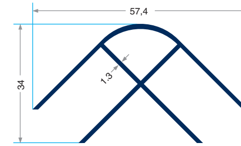
PRV-6110 532 gr/m Açılı Bağlı Dikme
