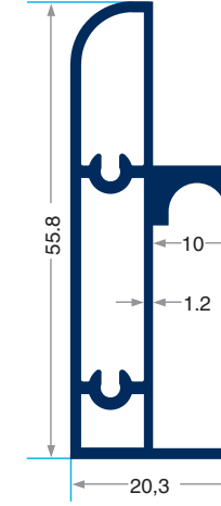
PRV-6013 642 gr/m Ray Profili
