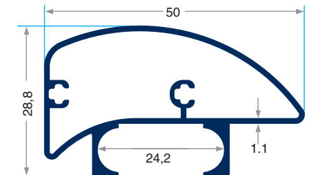
PRV-6023 558 gr/m RayProfili
