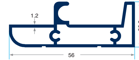
PRV-6161 628 gr/m Ray Profili
