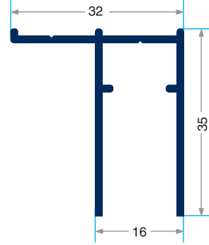
PRV-6030 342gr/m Duvar Dikme
