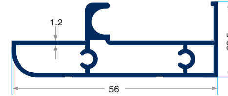
PRV-6162 607 gr/m Ray Profili
