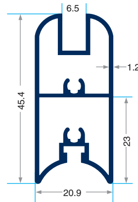
PRV-6280 640 gr/m Cam Dikmesi
