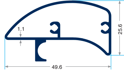
PRV-6160 516gr/m Lüks SeriRay
