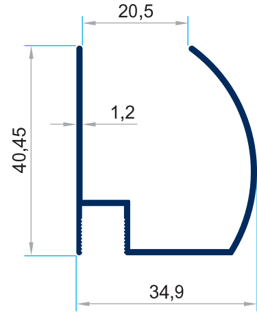
PRV-6140 392 gr/m Lüks Seri Cam U
