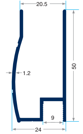
PRV-6141 410 gr/m Cam U Profili
