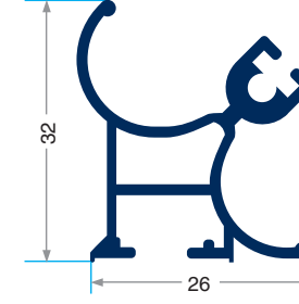
PRV-6090 431gr/m Köşe Kirişli Dikme
