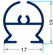
PRV-6070 221 gr/m Orta Dikme
