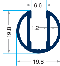
PRV-6290 287 gr/m Menteşe Profili
