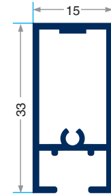
PRV-6040 308gr/m Askılık
