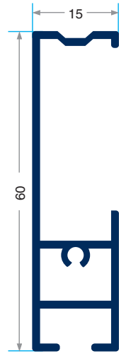
PRV-6010 441gr/m Jakuzi Dış Ray
