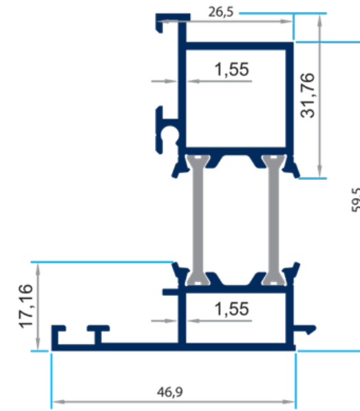
PRV-4724 1.040 g r/m Çeyrek S erikasa
