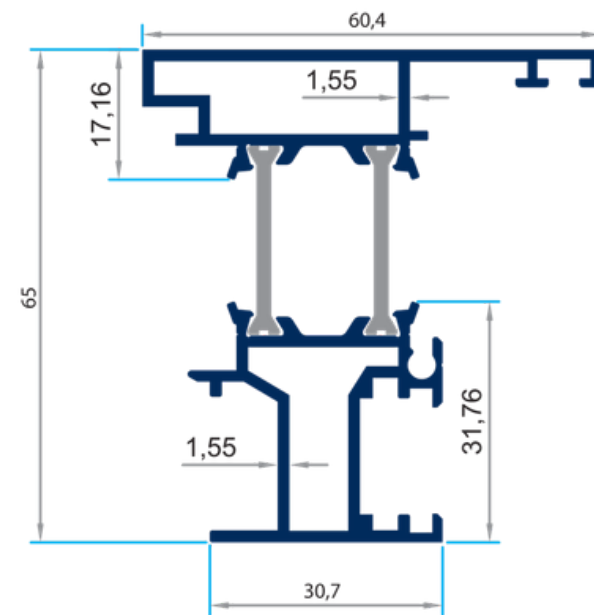
PRV-4723 1.285gr/m Kanat A daptörü
