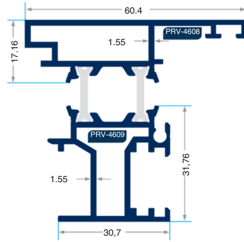
PRV-4610 1.285 gr/m Kanat A adaptörü
