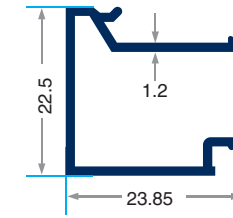
PRV-4670 259 gr/m Isı Cam Çitası 20 mm
