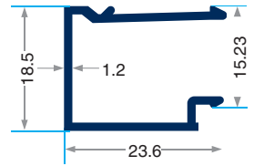
PRV-4671 232 gr/m Isı Cam Çitası 24 mm
