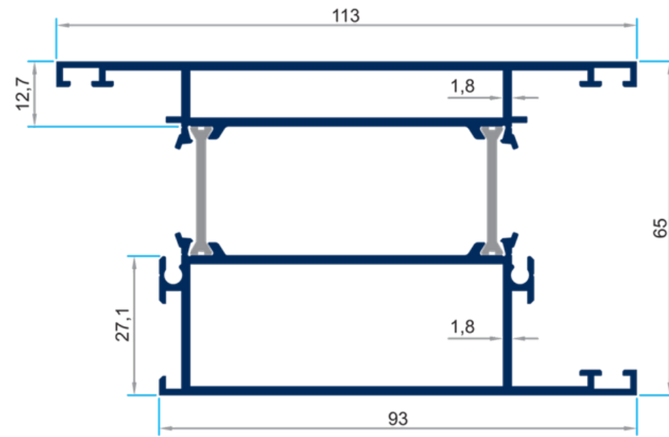
PRV-4722 2.300gr/m EtekProfili
