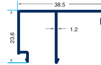
PRV-4650 312 gr/m Tek CamÇitası
