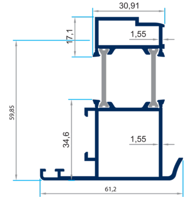
PRV-4725 1.240 g r/m Pivot A daptörü
