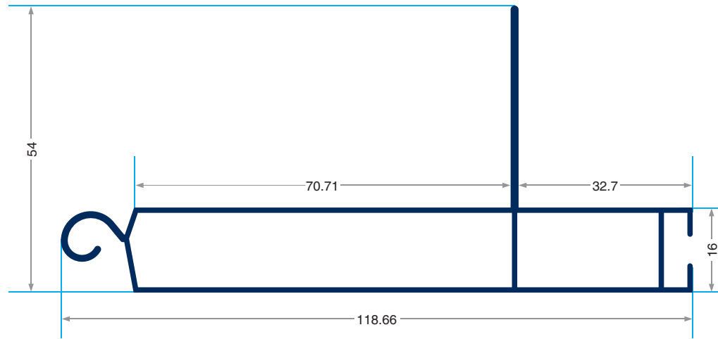
PRV-1561 950gr/m Kepenik Alt Etek
