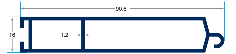
PRV-1560 726 gr/m Kepenik Alt Etek
