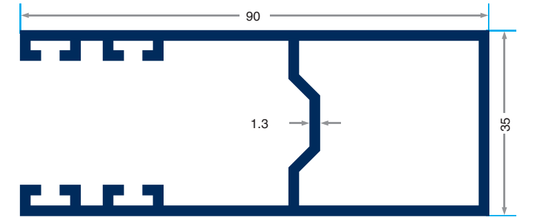
PRV-1550 1103 gr/m 90'lik Yan U
