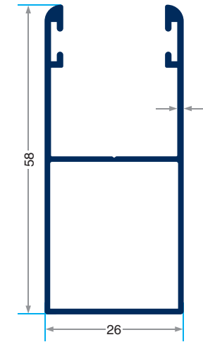
PRV-1591 502 gr/m Panjur Yan Ray
