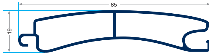
PRV-1520 515gr/m 77'likLamel
