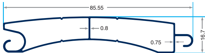
PRV-1521 475gr/m 77'likLamel
