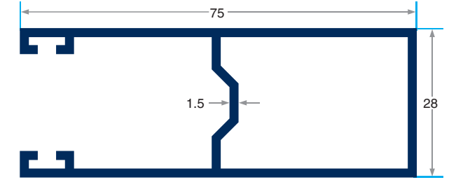
PRV-1540 910 gr/m 75'lik Yan U
