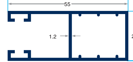
PRV-1530 600 gr/m Panjur Yan U
