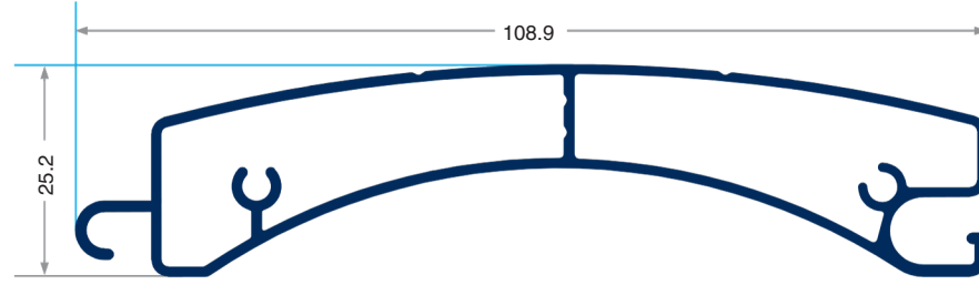
PRV-1510 955gr/m 100'likLamel
