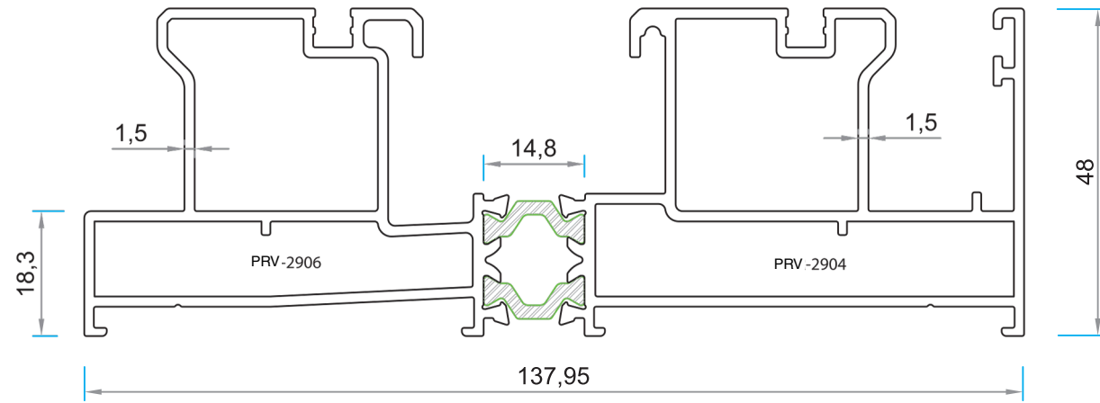
PRV-2942 Ağırlık (kg/mt): 2,678 STATİK / STATIC Jx (cm 4 ): 22,47 Jy (cm 4 ): 163,85
