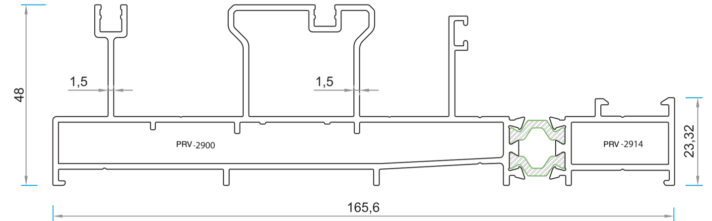
PRV-2945 Ağırlık (kg/mt): 2,646 STATİK / STATIC Jx (cm 4 ): 17,20 Jy (cm 4 ): 214,04
