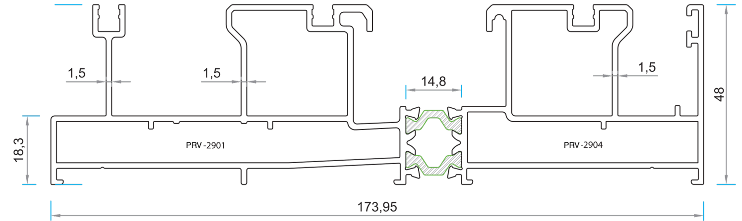
PRV-2943 Ağırlık (kg/mt): 3,191 STATİK / STATIC Jx (cm 4 ): 22,47 Jy (cm 4 ): 163,85
