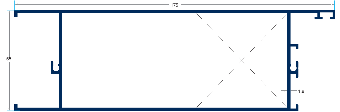
PRV-5520 2263 gr/m 175'lik Etek
