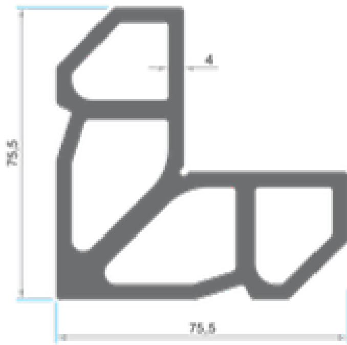
PRV-5506 4,241 gr/m Köşe T akozu
