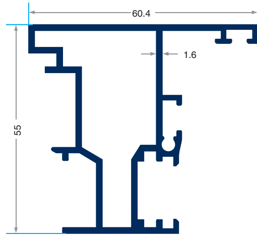
PRV-5530 1127 gr/m Kanat A daptörü
