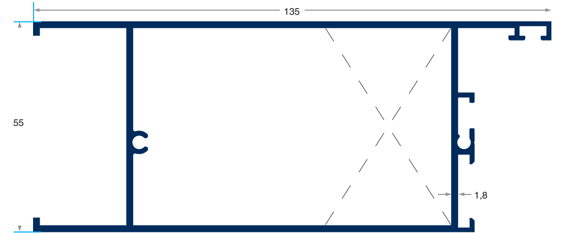
PRV-5521 1867 gr/m 135'lik Etek
