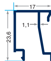
PRV-5519 222 gr/m 24 mm lisi Cam Çitisi
