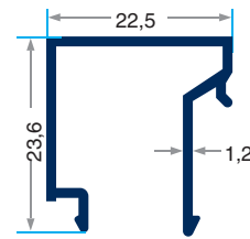
PRV-4670 257 gr/m 20 mm lisi Cam Çitisi
