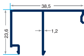
PRV-4650 312 gr/m 6 mm Tek Cam Çitisi
