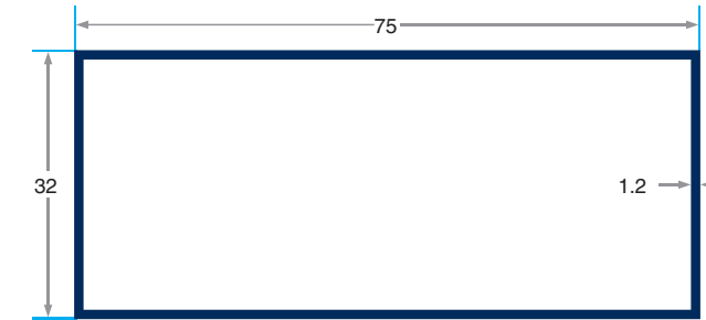
PRV-9530 680 gr/m 32x75 Kutu Profili
