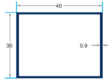
PRV-2580 332 gr/m 30x40 Kutu Profili
