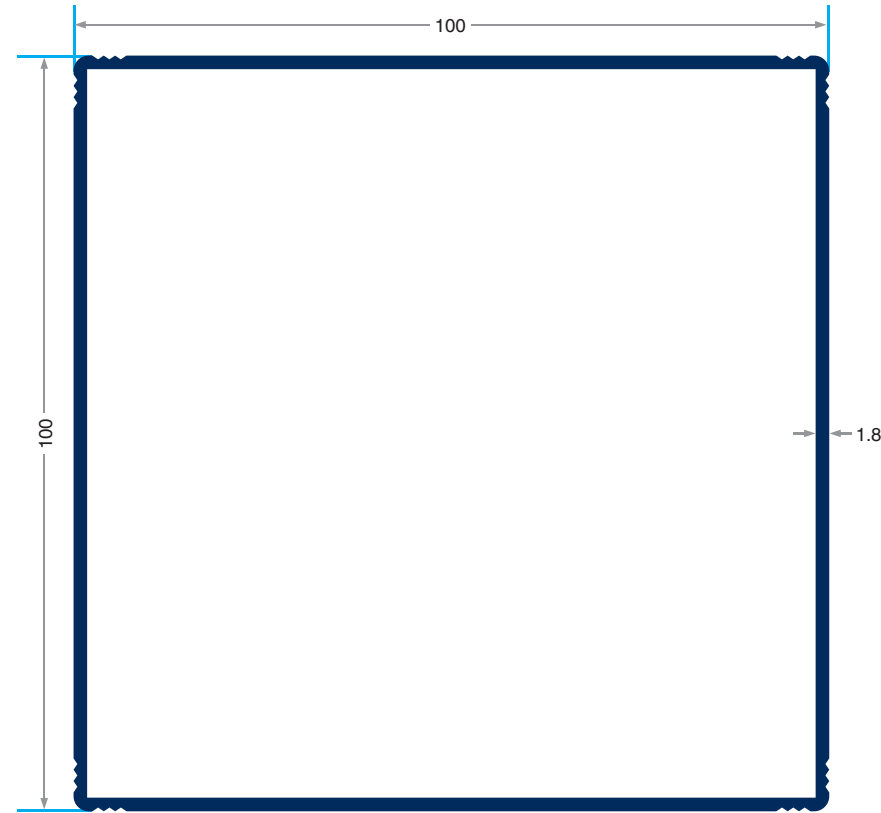
PRV-4413 1.182 gr/m 100 x 100 Kutu Profili
