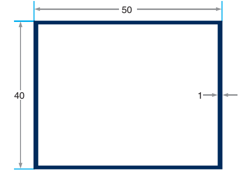
PRV-9540 477 gr/m 40x50 Kutu Profili
