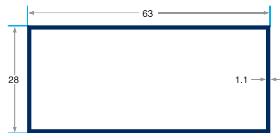
PRV-9520 482 gr/m 28x63 Kutu Profili
