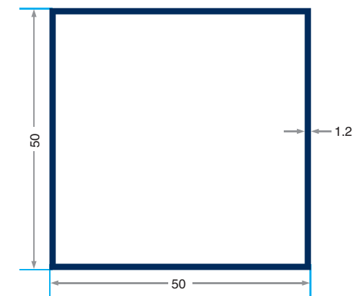
PRV-9781 634 gr/m 50x50 Kutu Profili
