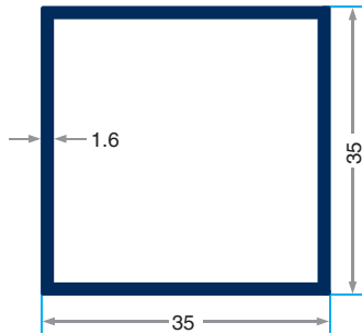
PRV-9592 579 gr/m 35x35KutuProfili
