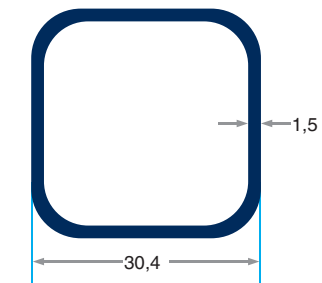
PRV-9640 434 gr/m 30'luk Boru 1.5 mm
