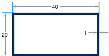
PRV-9510 314 gr/m 20x40KutuProfili
