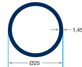
PRV-9620 291 gr/m 25'lik Boru 1.6 mm
