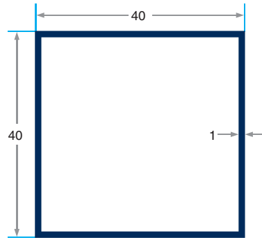
PRV-2520 421 gr/m 40x40 Kutu Profili
